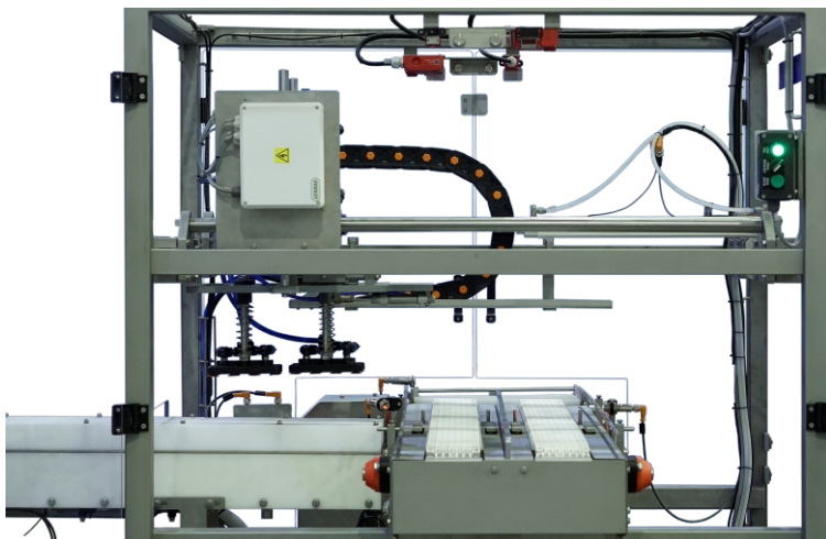
. Encajonador automático incorporado . Built-in automated case-packer
