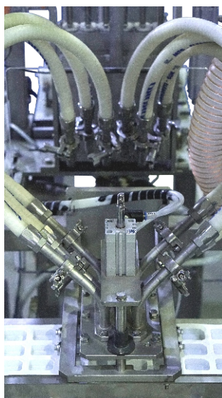
Opcional Dosificador servoactuated Optional Servo-driven filler
