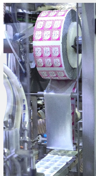
Opcional Desinfección UV en film de lamina de tapa Optional UV light in lid film unwinder
